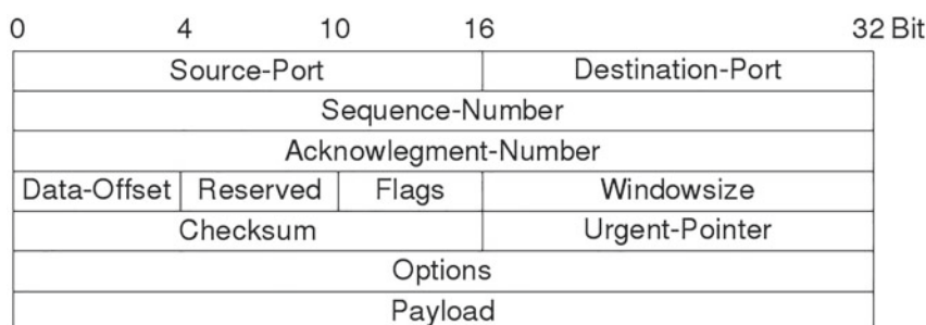
Fig. 2.11 TCP-Header
