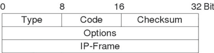
Fig. 2.10 ICMP-Header
